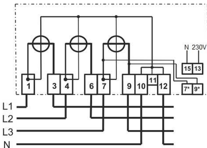
Abb. 2: Anschlussschaltbild 4102 mit Zusatzklemmen
