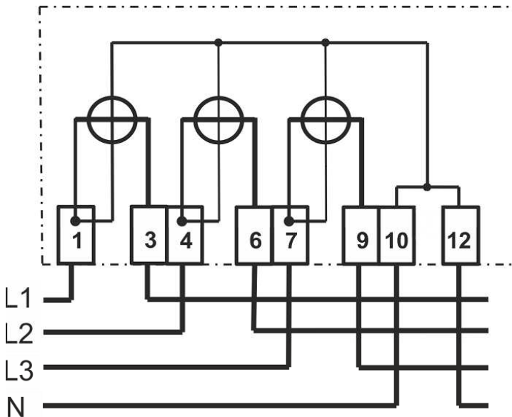
Abb. 1: Anschlussschaltbild 4100 ohne Zusatzklemmen
