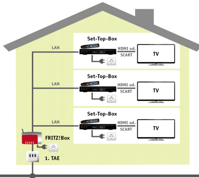
Hauszuführung „Bestehender Telefon-Hausanschluss“ oder Hauszuführung Glasfaserkabel Stadtwerke OELS NITZ/V. GmbH
